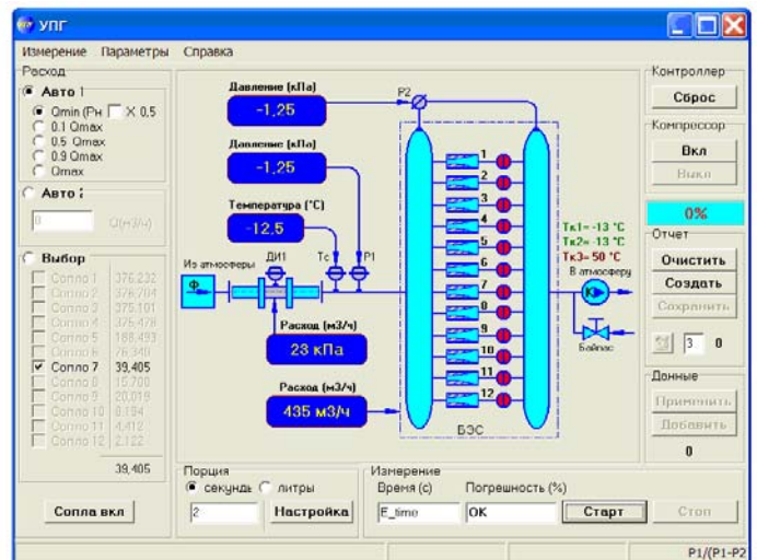
УСТАНОВКА ПОВЕРОЧНАЯ ГАЗОВАЯ УПГ. МНМОСХЕМА
